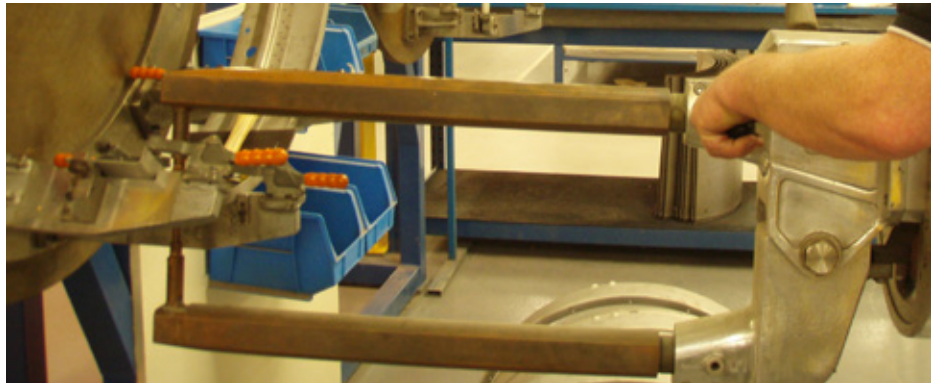
Figura 7.2. Equipo de soldadura por puntos suspendido portátil
