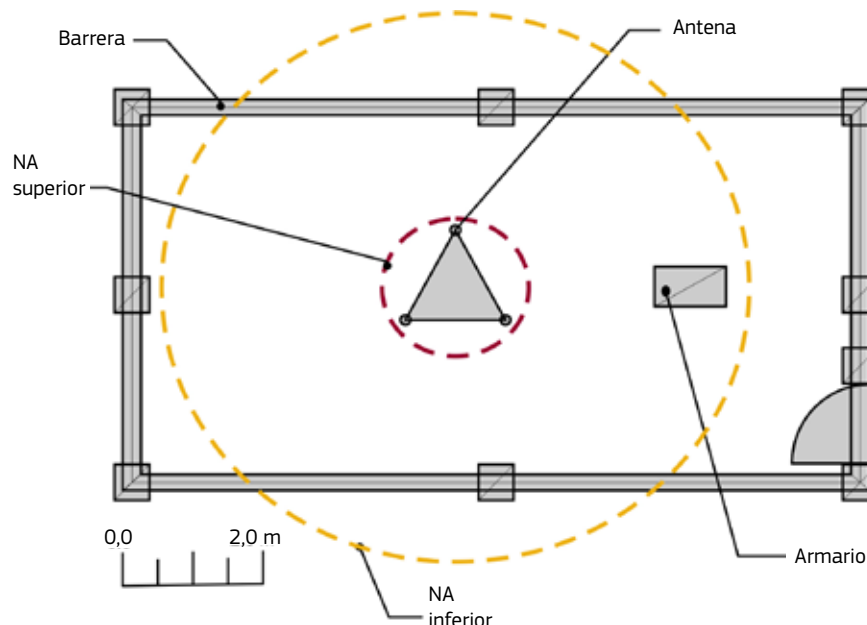
Figura 12.3. Vista en planta que muestra los contornos dentro de los cuales podrían superarse los niveles de actuación en torno al radiofaro no direccional
