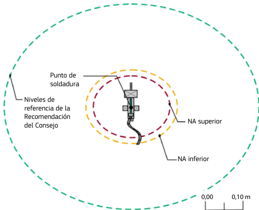
Figura 6.20. Vista en planta que muestra los contornos dentro de los cuales podrían superarse el nivel de actuación inferior (amarillo) y el nivel de actuación superior (rojo) en torno a la pistola de soldar por puntos de «tipo X» de 700 mm de la fábrica. En este caso, los contornos se extienden por detrás de la pistola debido a campos creados por conductores de la parte posterior de la misma
